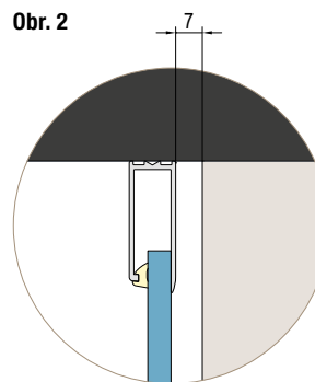
Bočná stena / fixný diel
